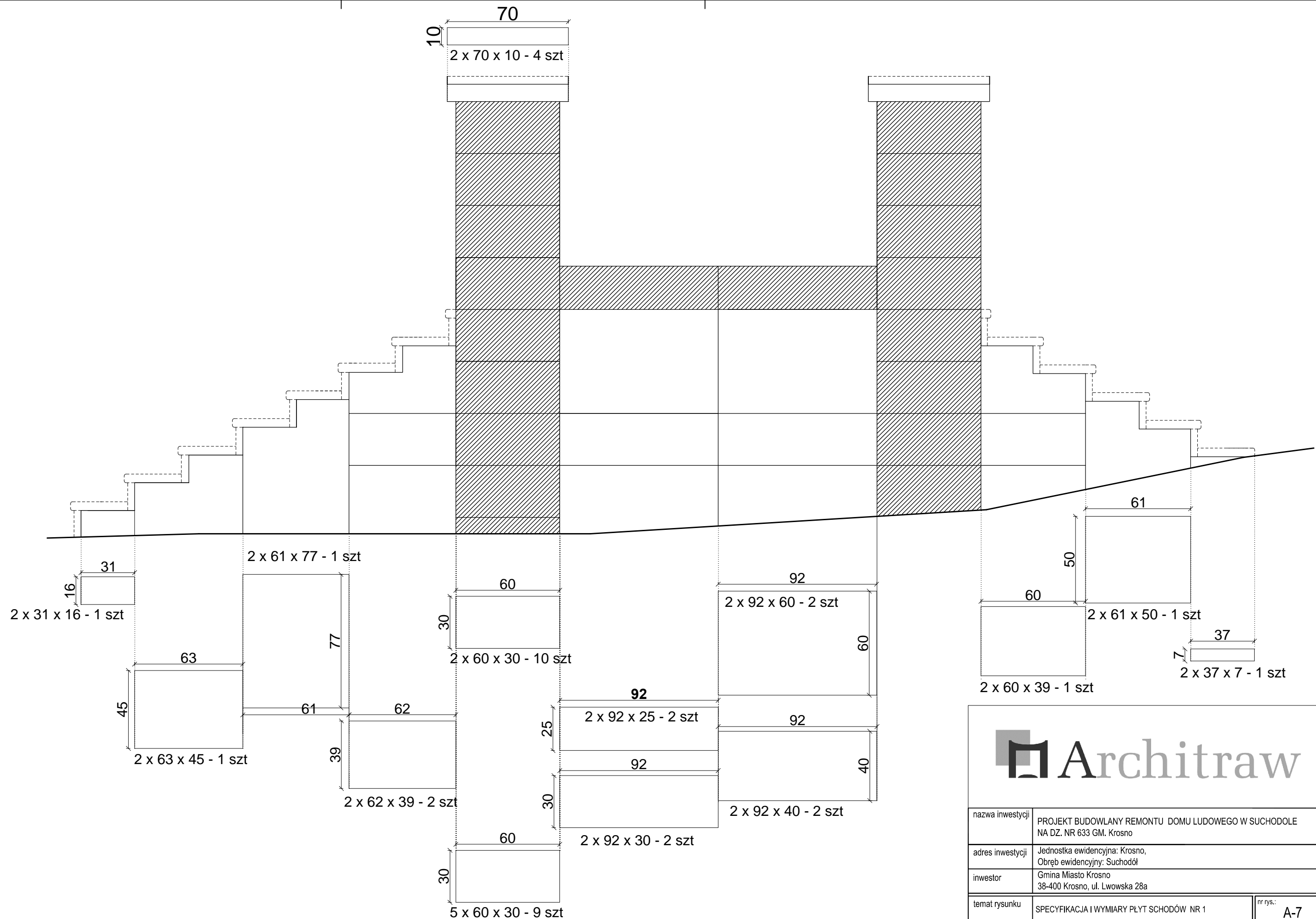
SPECYFIKACJA I WYMIARY PŁYT PIASKOWYCH - WIDOK SKALA 1:20
