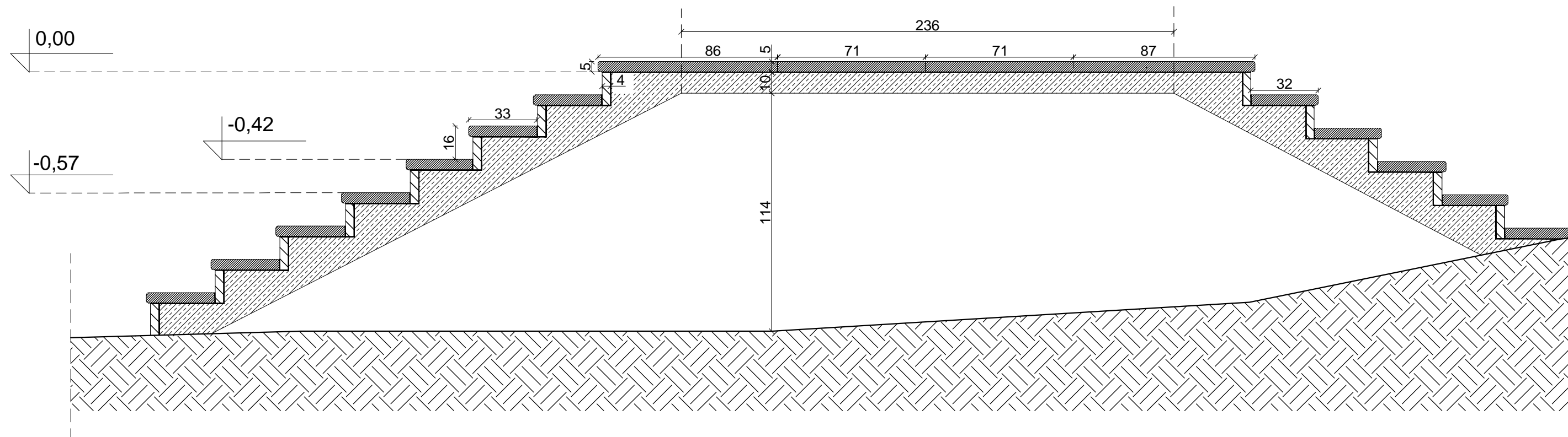
PRZEKRÓJ C-C PRZEZ GŁÓWNE SCHODY SKALA 1:20
