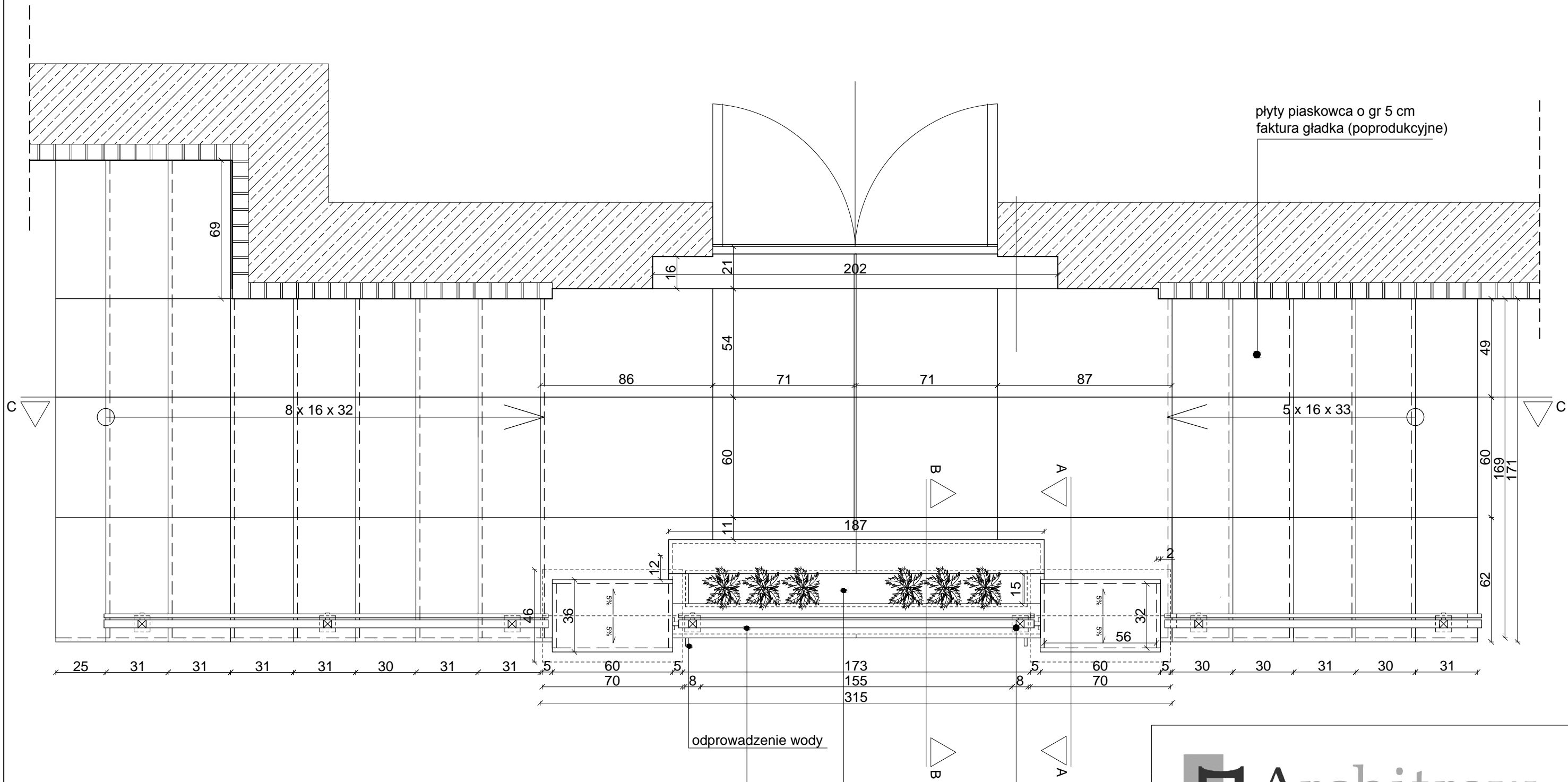
RZUT SCHODÓW nr 1 - GŁÓWNE WEJŚCIE DO BUDYNKU SKALA 1:20
